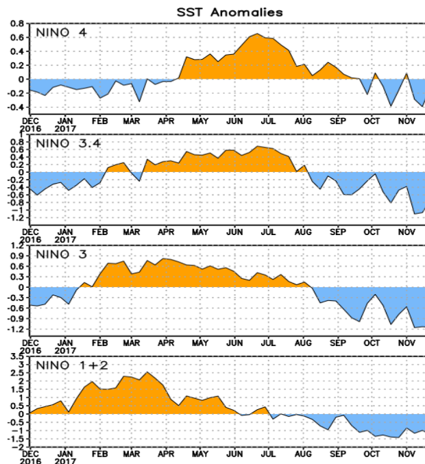
Figura 2. Series de Tiempo de las anomalías (en °C) de temperaturas de la superficie del océano (TSM) en un área promediada en las regiones de El Niño [Niño-1+2 (0°-10°S, 90°W-80°W), Niño 3 (5°N-5°S, 150°W-90°W), Niño-3.4 (5°N-5°S, 170°W-120°W), Niño-4 (150°W-160°E y 5°N-5°S)]. Las anomalías de temperatura de la superficie del océano son variaciones de los promedios semanales del período base de 1981-2010.
