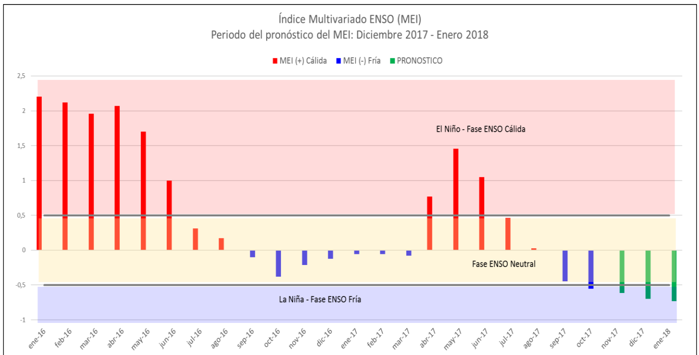
Gráfica 1. Registros del Índice Multivariado del ENOS (MEI,) para el periodo de enero de 2016 a agosto de 2017 y sus respectivos pronósticos para los meses de septiembre a diciembre 2017.
